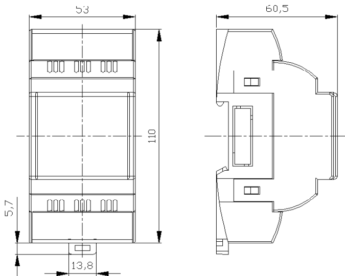
Rysunek 2. Wymiary miernika.
