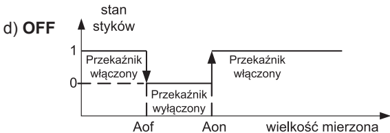
Rys 9. Typy alarmów: a) n-on ,b) n-oFF c) On d) OFF.
