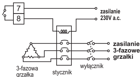
Rys.33. Wyjście typu przekaźnik do sterowania stycznikiem trójfazowym
