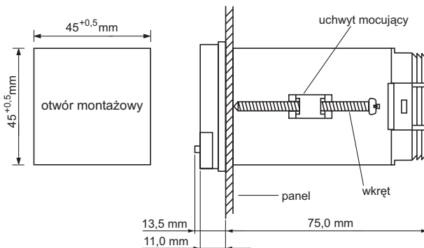
Rys.7. Mocowanie regulatora.
