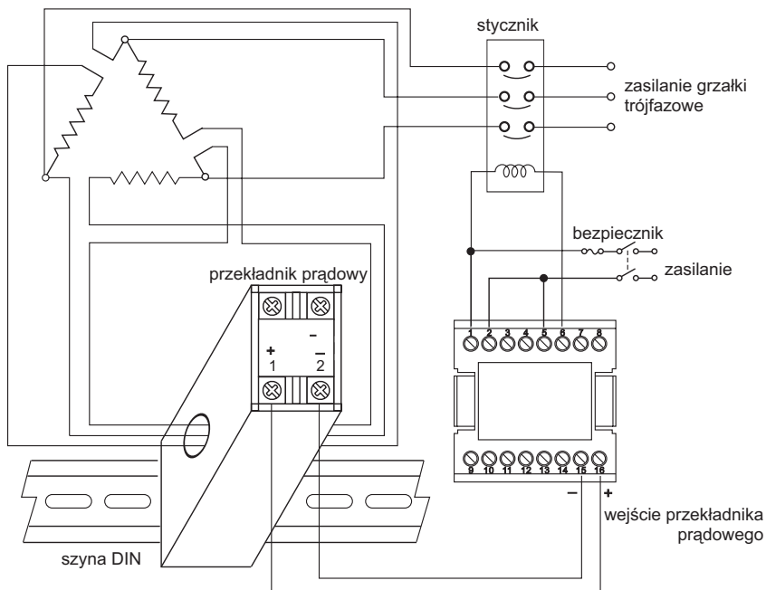
Rys.18. Podłączenie przekładnika prądowego do grzałki trójfazowej
