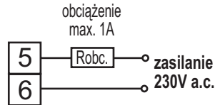
Rys.25. Wyjście typu triak do bezpośredniego sterowania obciążeniem
