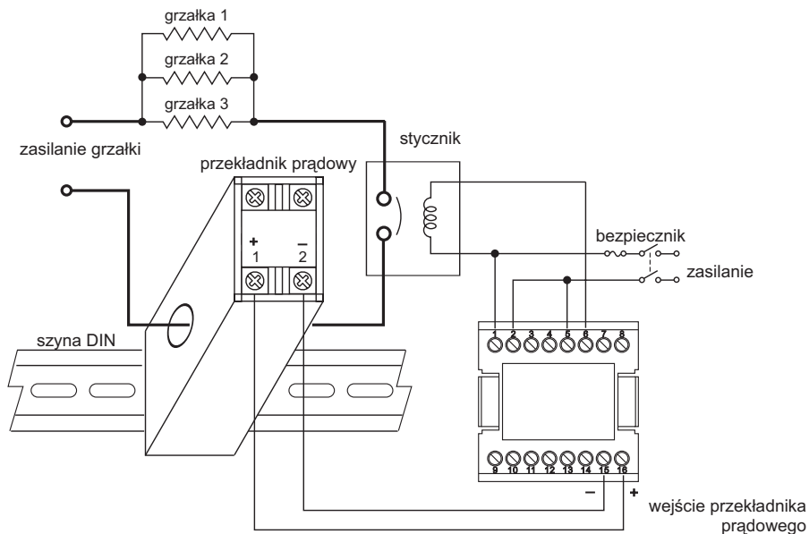
Rys.17. Podłączenie przekładnika prądowego do grzałki jednofazowej
