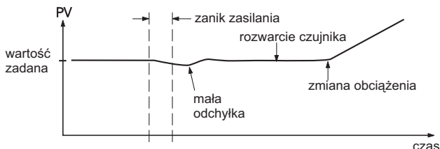
Rys.61. Praca regulatora w trybie awaryjnym z przelączeniem bezuderzeniowym.
