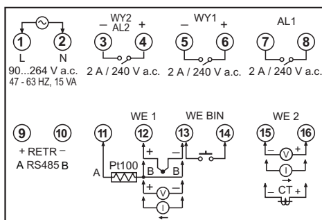
Rys.9. Opis listwy zaciskowej.
