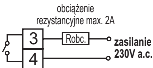
Rys.26. Wyjście typu przekaźnik do bezpośredniego sterowania obciążeniem
