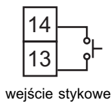
Rys.19. Podłączenie wejścia binarnego
