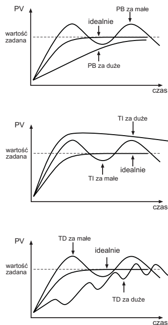
Rys.66. Efekty doboru nastaw PID.
