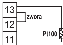
Rys.12. Podłączenie Pt100.
