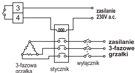
Rys.35. Wyjście typu przekaźnik do sterowania stycznikiem trójfazowym
