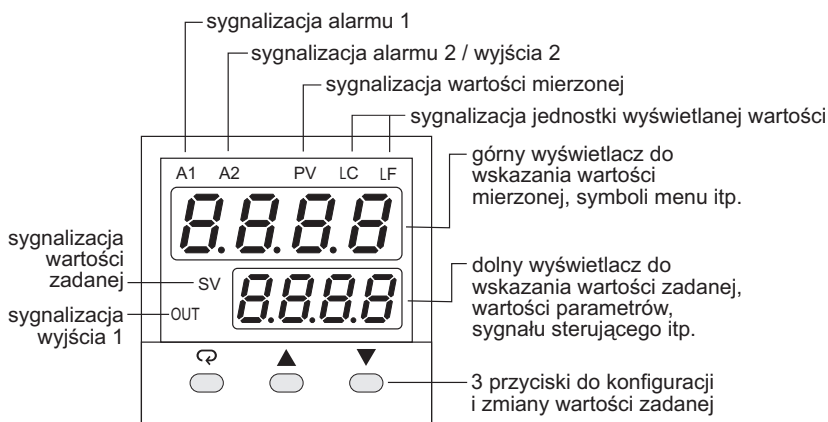
Rys.3. Opis panelu przedniego.
