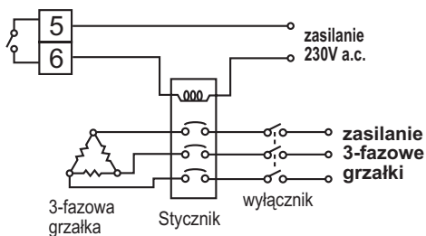
Rys.21. Wyjście typu triaik lub triaik do sterowania stycznikiem trójfazowym
