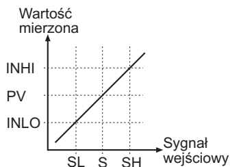
Rys.40. Wykres przekształcenia sygnału analogowego na wskazanie
