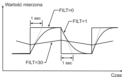
Rys.74. Filtr cyfrowy
