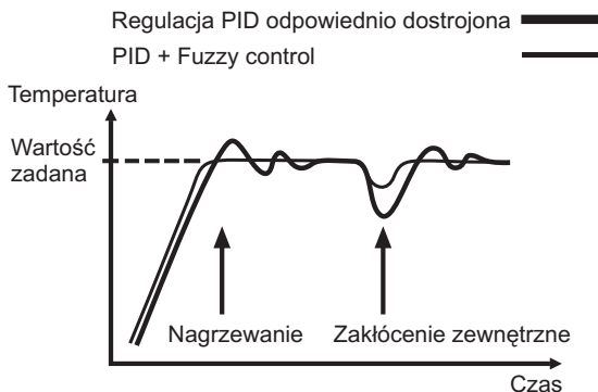
Rys.1. Korzyści z zastosowania funkcji fuzzy-logic.
