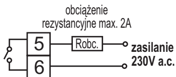
Rys.20. Wyjście typu przełącznik do bezpośredniego sterowania obciążeniem
