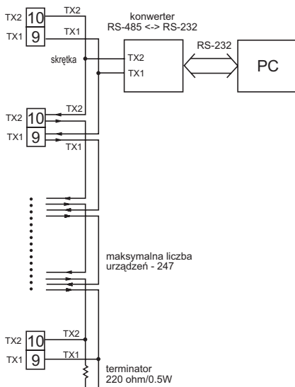
Rys.36. Podłączenie RS-485
