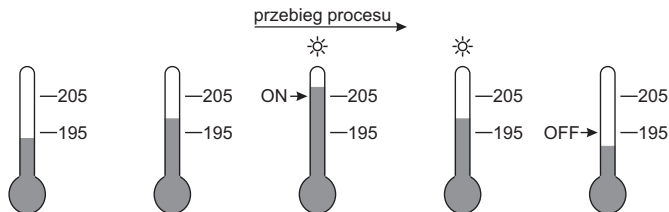
Rys.44. Alarm bezwzględny normalny.
