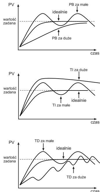
Rys.66. Efekty doboru nastaw PID.
