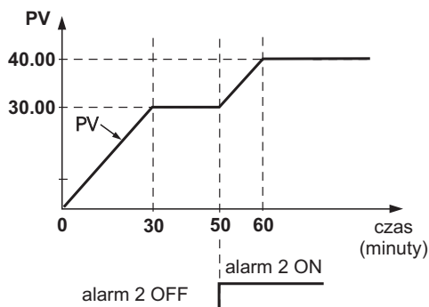
Rys.70. Program narostu i wygrzewania.
