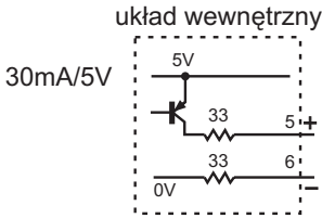
Rys. 22. Wyjście napięciowe 0/5V do sterowania przełącznika półprzewodnikowego (SSR)
