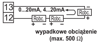
Rys.37. Wyjście retransmisyjne prądowe
