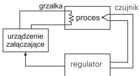
Rys.57. Źródła przerwania pętli regulacji.
