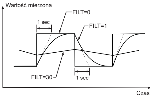
Rys.74. Filtr cyfrowy
