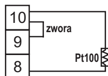
linia 2-przewodowa
