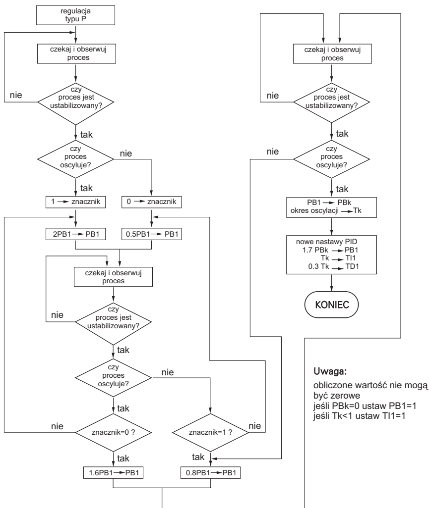
Rys.64. Ręczny dobór parametrów PID.
