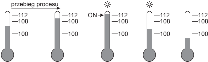
Rys.49. Alarm względny z pamięcią.
