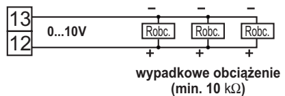
Rys.38. Wyjście retransmisyjne napięciowe
