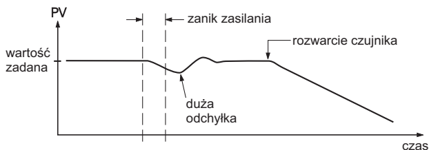
Rys.60. Praca regulatora w trybie awaryjnym bez przelączenia bezuderzeniowego.
