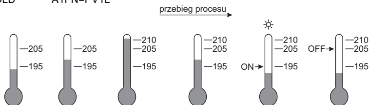
Rys.46. Alarm bezwzględny z wstrzymaniem.
