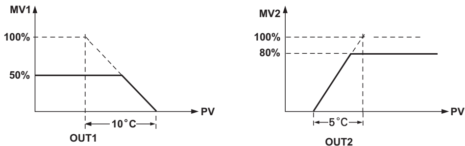
Rys.72. Ograniczenie sygnału sterującego.
