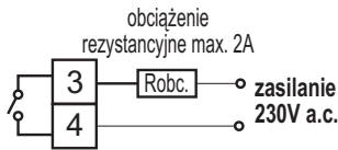
Rys.34. Wyjście typu przełącznik do bezpośredniego sterowania obciążeniem
