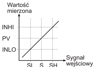
Rys.40. Wykres przekształcenia sygnału analogowego na wskazanie
