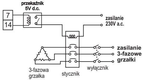
Rys.33. Wyjście napięciowe 0/5V do sterowania stycznikiem trójfazowym przez zewnętrznym przełącznikiem
