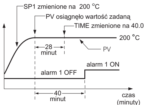
Rys.69. Timer czasu wygrzewania.
