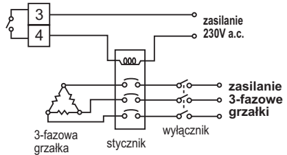
Rys.35. Wyjście typu przełącznik do sterowania stycznikiem trójfazowym
