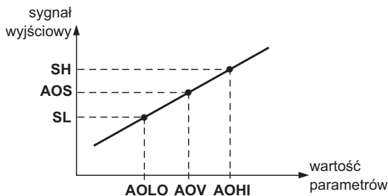
Rys.73. Sposób konwersji sygnału dla retransmisji.
