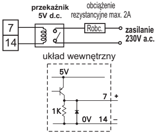
Rys.32. Wyjście napięciowe 0/5V do sterowania zewnętrznym przełącznikiem
