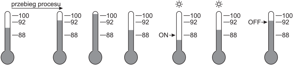
Rys.50. Alarm względny z wstrzymaniem.
