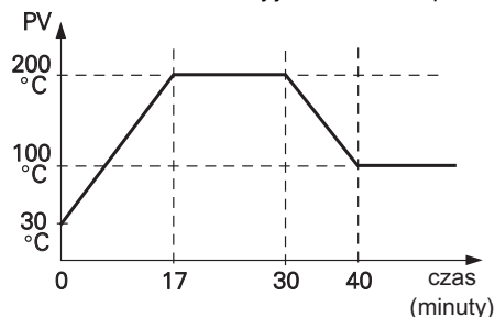
Rys.68. Funkcja miękkiego startu.
