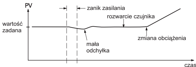
Rys.61. Praca regulatora w trybie awaryjnym z przelączeniem bezuderzeniowym.
