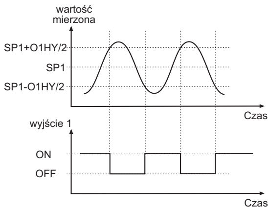
Rys.41. Regulacja załącz-wyłącz typu grzanie
