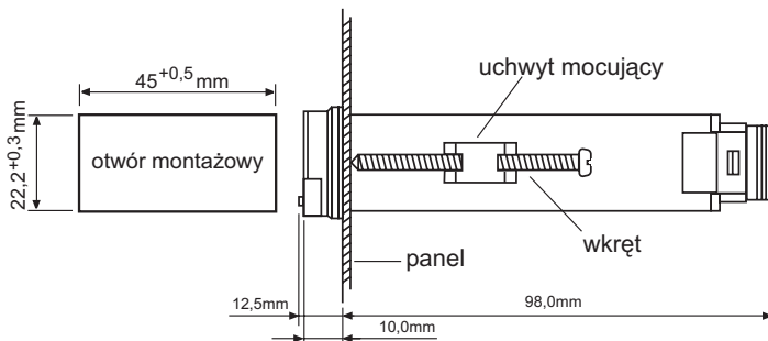
Rys.7. Mocowanie regulatora.
