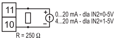
Rys.16. Podłączenie wejścia liniowego prądowego.
