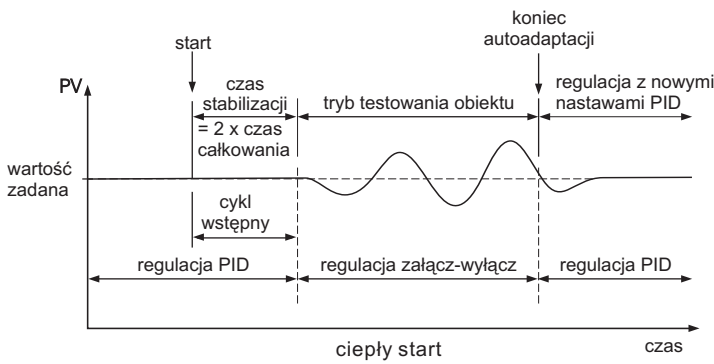
Rys.63. Autoadaptacja dla ciepłego startu.
