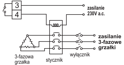
Rys. 27. Wyjście typu przełącznik lub triak (SSR) do sterowania stycznikiem trójfazowym
