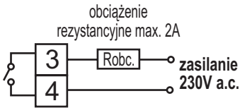
Rys. 26. Wyjście typu przełącznik do bezpośredniego sterowania obciążeniem
