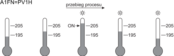
Rys.45. Alarm bezwzględny z pamięcią.
