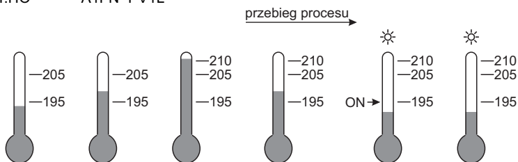
Rys.47. Alarm bezwzględny z pamięcią i wstrzymaniem.
