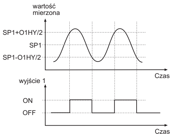
Rys.42. Regulacja załącz-wyłącz typu chłodzenie
