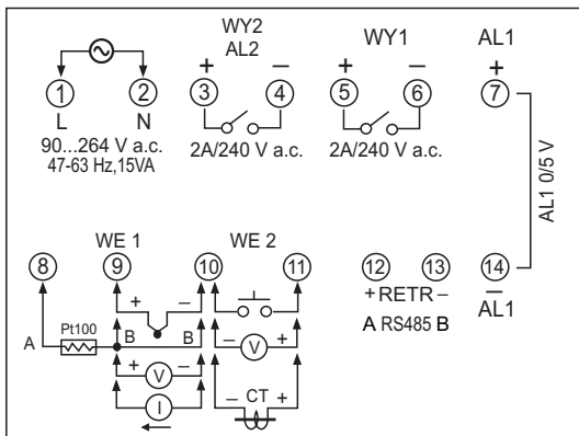
Rys.9. Opis listwy zaciskowej.
