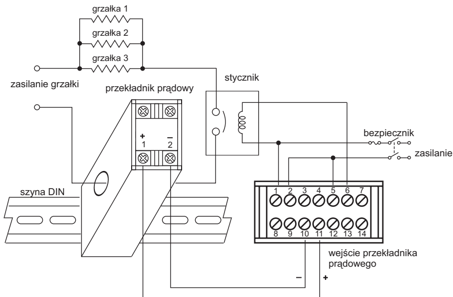
Rys.17. Podłączenie przekładnika prądowego do grzałki jednofazowej
