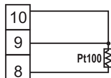
linia 3-przewodowa
