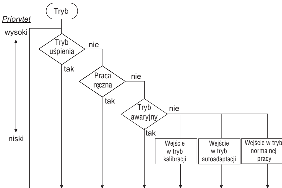
Rys.6. Priorytet trybów pracy.
