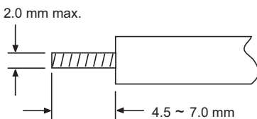
Rys.8. Wymiary końcówek przewodów podłączanych do listwy zaciskowej.
