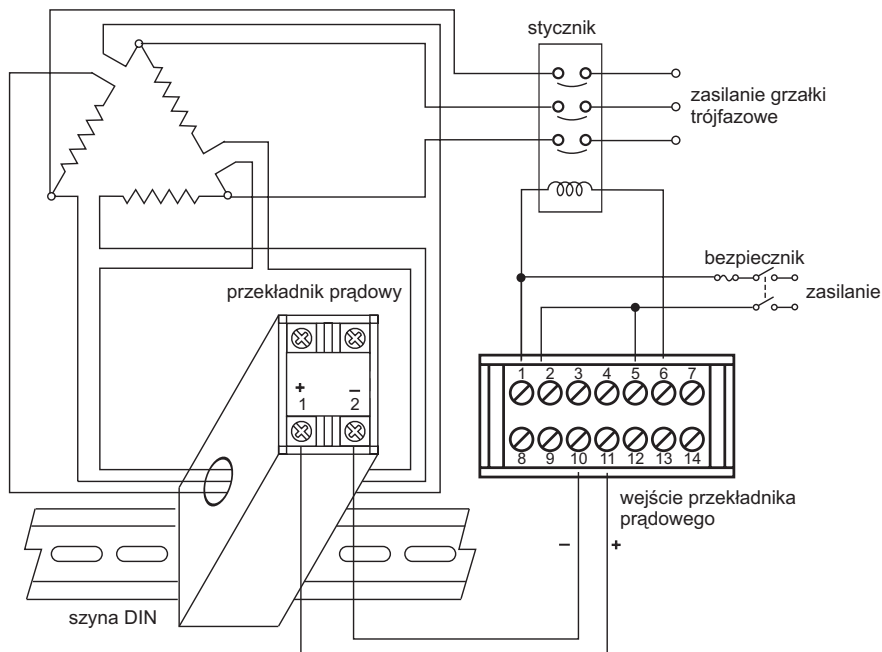
Rys.18. Podłączenie przekładnika prądowego do grzałki trójfazowej
