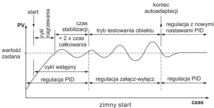
Rys.62. Autoadaptacja dla zimnego startu.
