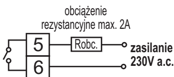
Rys.20. Wyjście typu przekaźnik lub triak (SSR) do bezpośredniego sterowania obciążeniem
