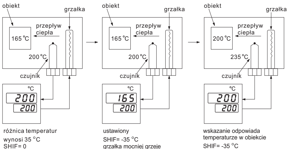
Rys.59. Zastosowanie przesunięcia wartości mierzonej.
