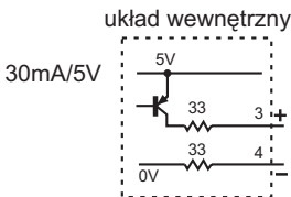
Rys. 28. Wyjście napięciowe 0/5V do sterowania przełącznika półprzewodnikowego (SSR)
