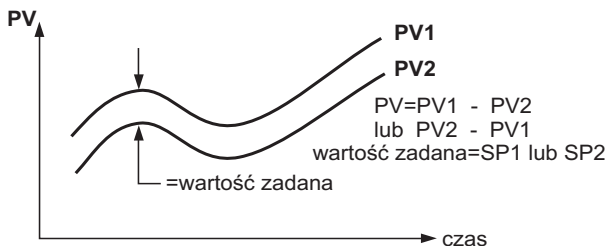
Rys.71. Zależności pomiędzy PV1 i PV2 w regulacji różnicowej.
