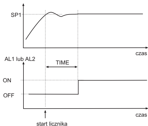
Rys.43. Funkcja timera czasu wygrzewania.
