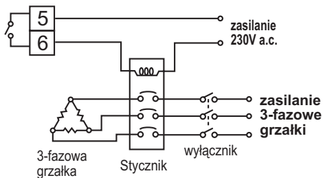
Rys.21. Wyjście typu przekaźnik lub triak (SSR) do sterowania stycznikiem trójfazowym
