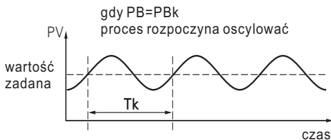
Rys.65. Stan na granicy stabilności.
