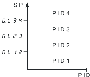
Rys. 19. „Gain Scheduling” przełączany od \mathcal{S} \mathcal{P}
