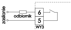
wyjście 3 - przekaźnik
