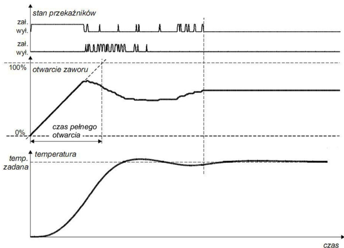
Rys. 18. Regulacja trójstawną krokowa bez sygnału zwrotnego
