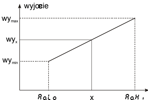
Rys. 24. Przeliczenie sygnału do retransmisji
