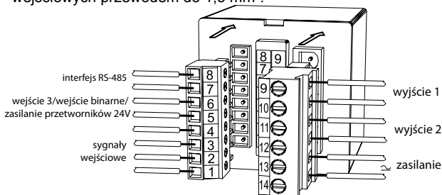
Rys. 3. Widok listew podłączeniowych regulatora.
