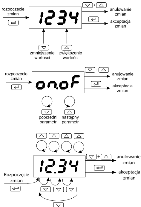
Rys. 15. Zmiana nastawy parametrów liczbowych i tekstowych.
