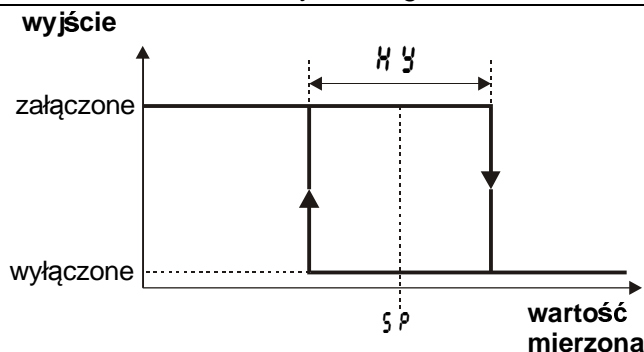
Rys. 13. Sposób działania wyjścia typu grzanie dla regulacji załącz-wyłącz
