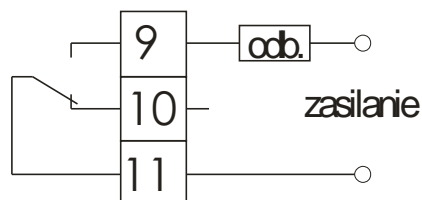
Rys. 6. Wyjście sterujące/alarmowe
