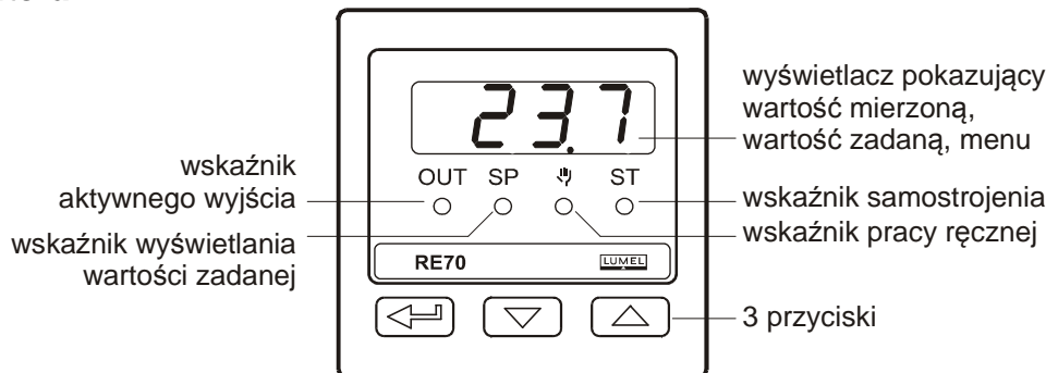
Rys. 8. Wygląd płyty czołowej regulatora.
