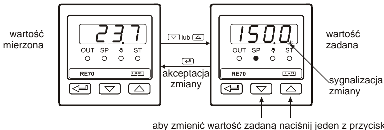
Rys. 9. Zmiana wartości zadanej.
