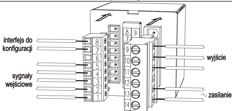
Rys. 3. Widok listew podłączeniowych regulatora.
