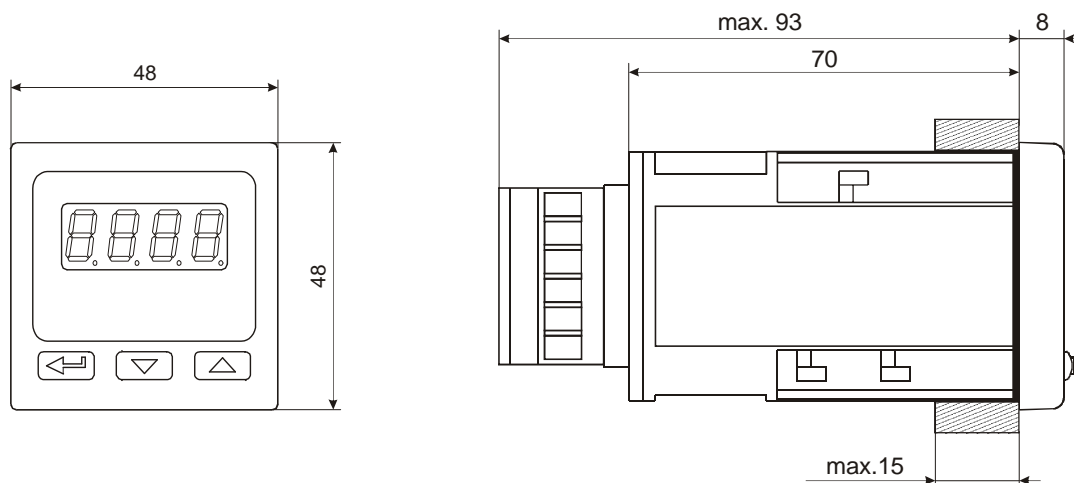
Rys. 2. Wymiary regulatora.
