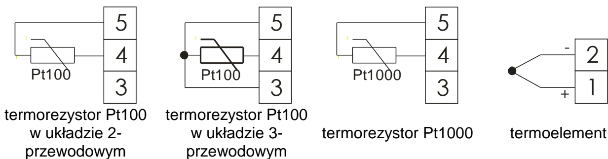
Rys. 4. Sygnały wejściowe
