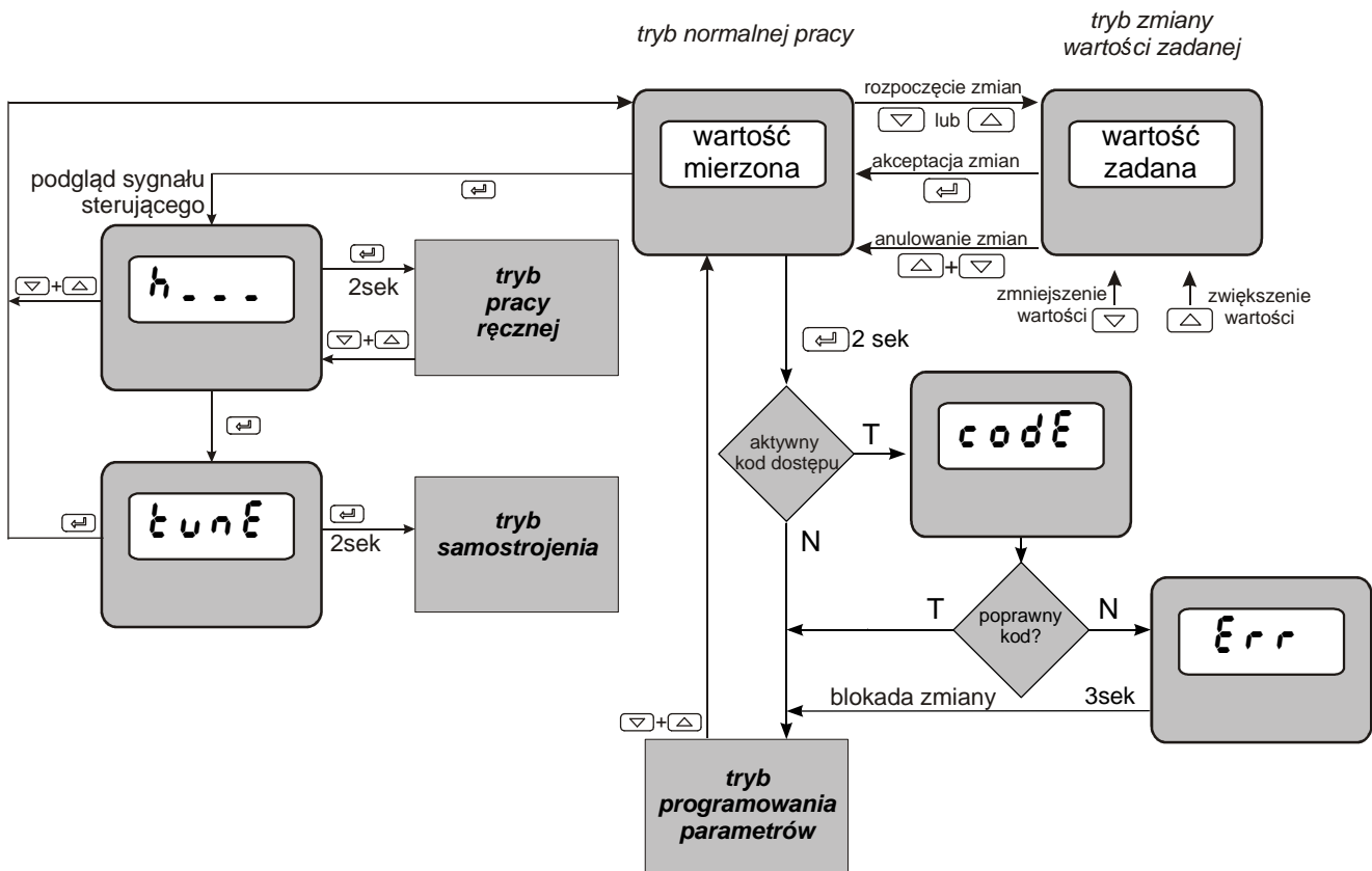
Rys. 10. Menu obsługi regulatora
