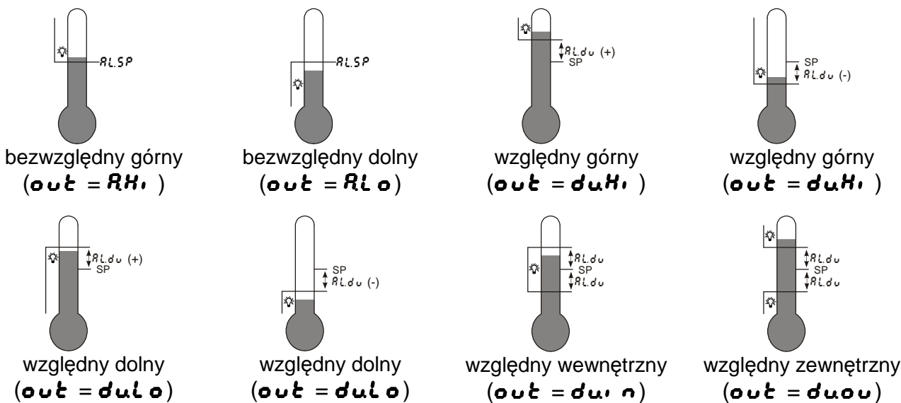
Rys.14. Rodzaje alarmów
